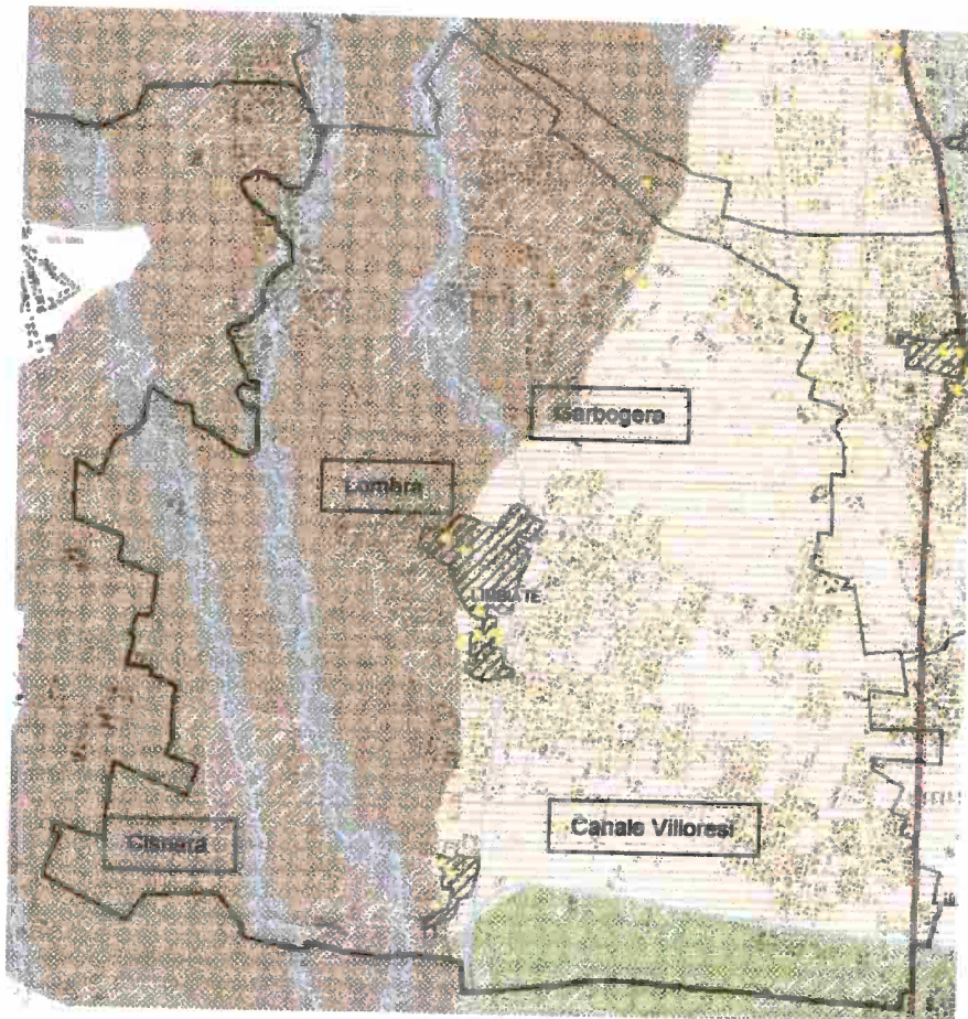
Figura 4: rete idrografica
