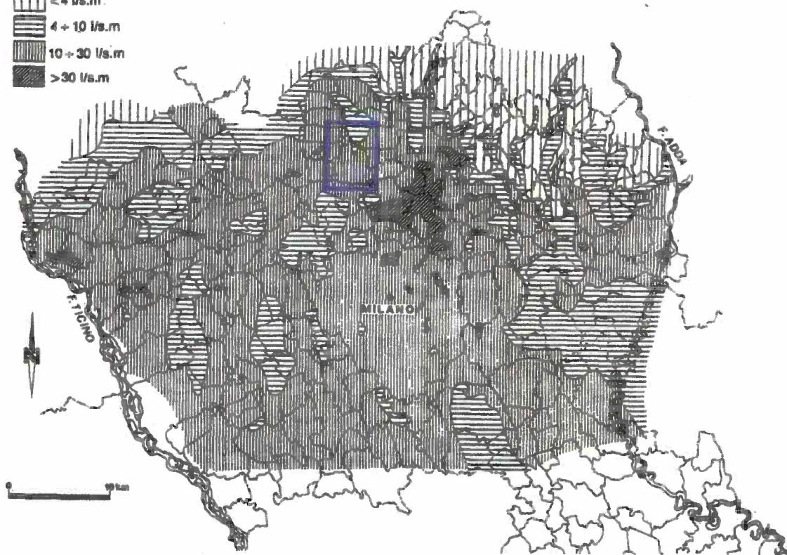
Fig. 20 — Carta della portata specifica.
