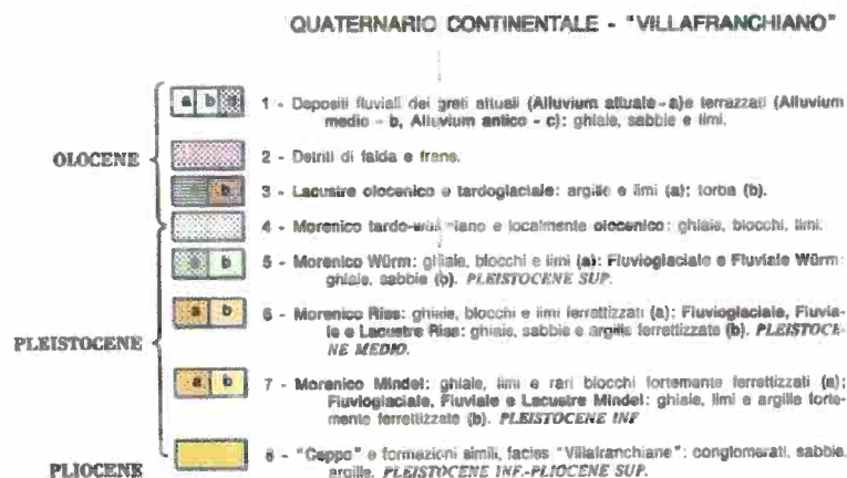
Figura 5: legenda della Carta Geologica
