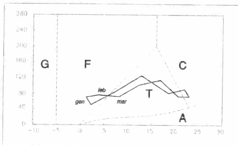
Figura 3: climogramma di Péguy (anni 1966-1997 - medie mensili)
