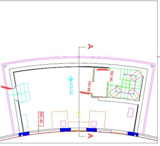
PIANTA CABINA
